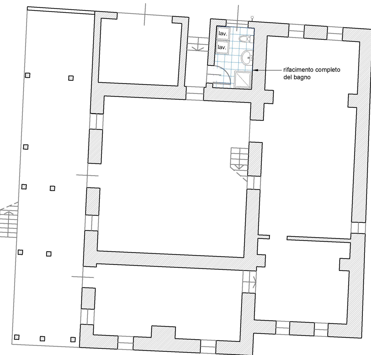
EDIFICIO A scala 1:100
